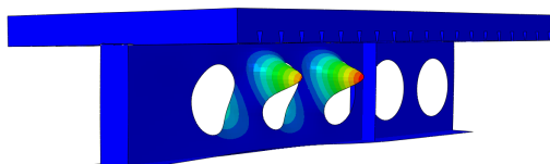
(d) CCB6: d/D_o=0.9 , p/D_o=1.4 , b_{wel}/b_w=3.8
