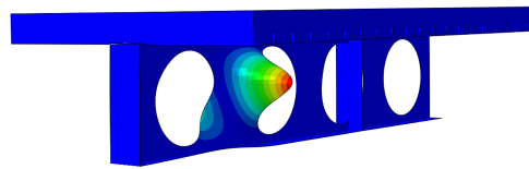
(d) CCB5: d/D_o=1.2 , p/D_o=1.5 and b_{we}/b_w=1.0
