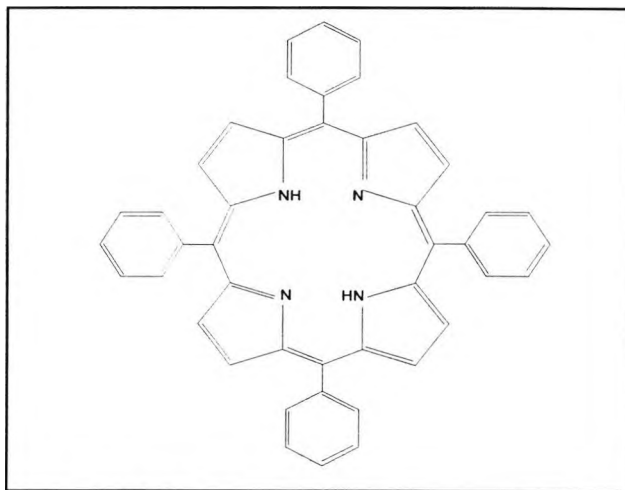
Fig. 1.7 - TPP
