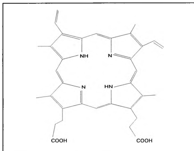
Fig. 1.6 - Protoporphyrin IX
