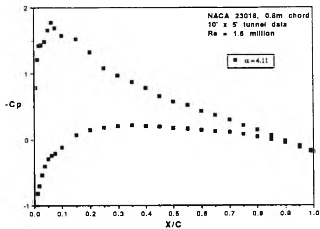
NACA 23018 aerofoil
