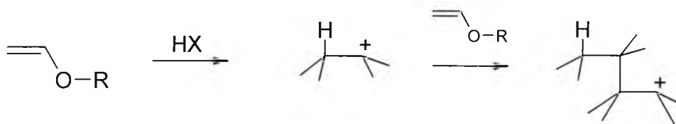
Scheme 3.3-10 Cationic polymerisation of a DVE
