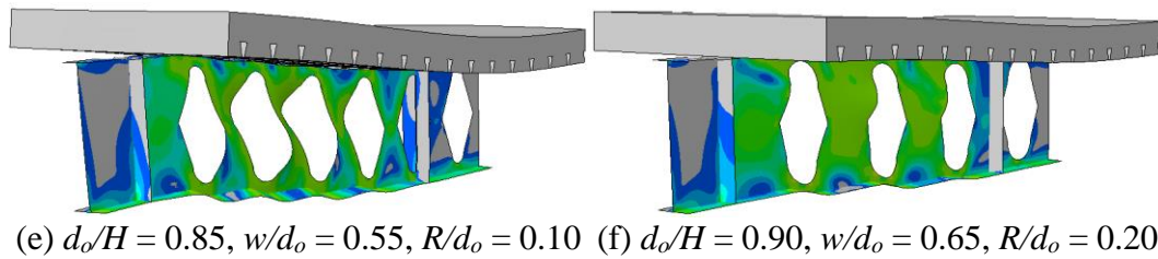
65 Fig. 14: WPB (Von Mises stresses in MPa), GCCB1.
