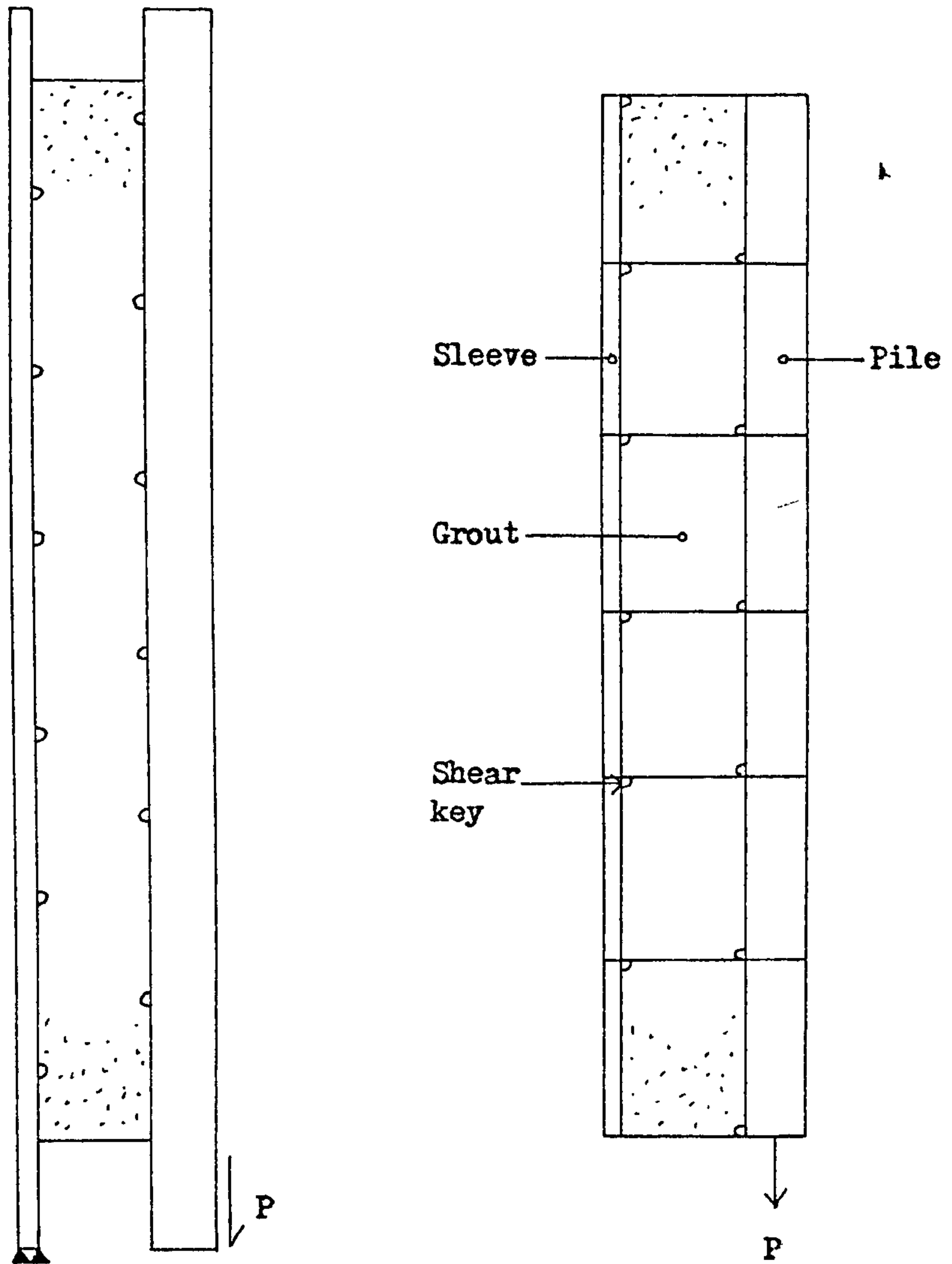
(a)Actual test
