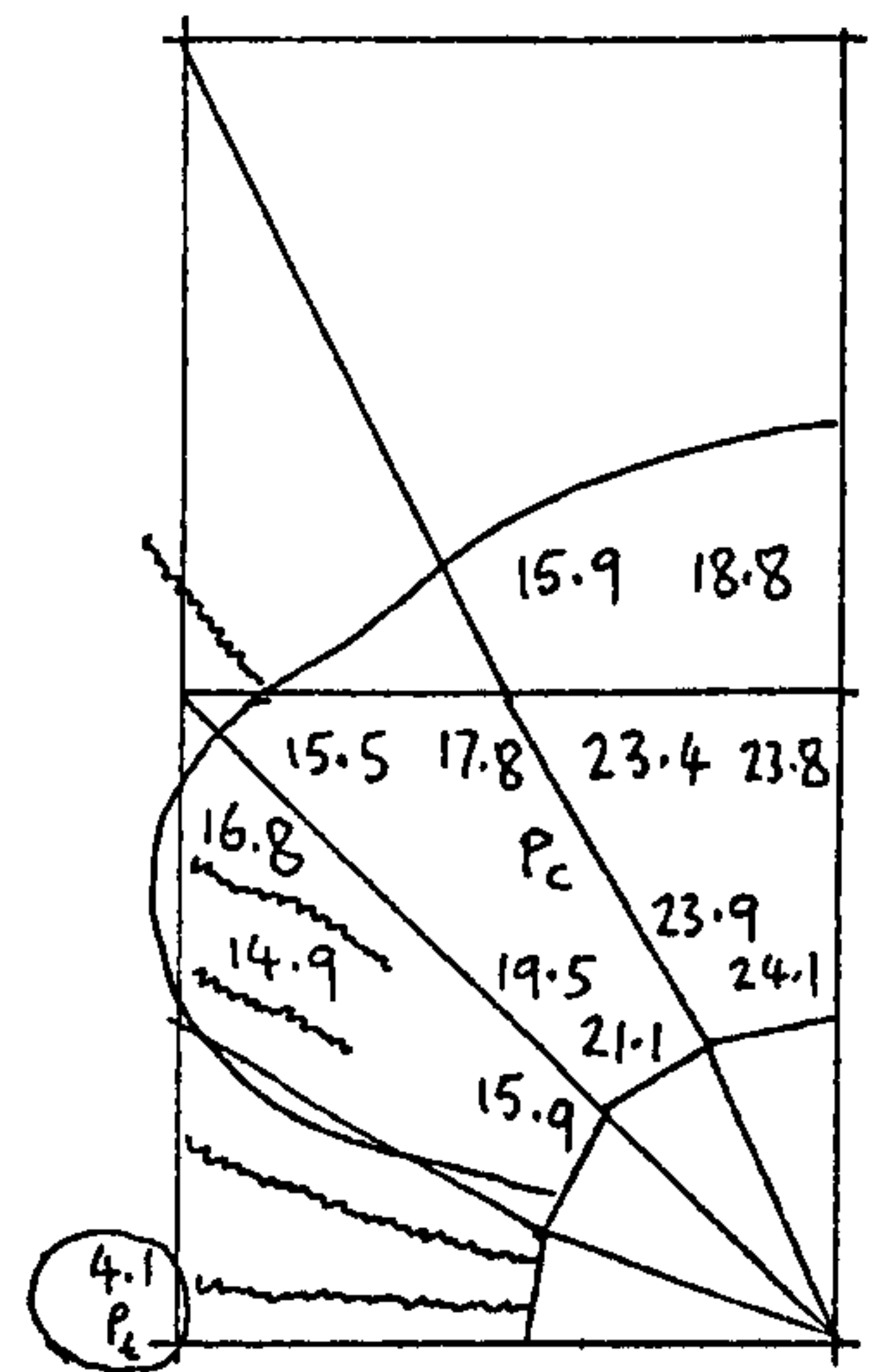
Load step 48
