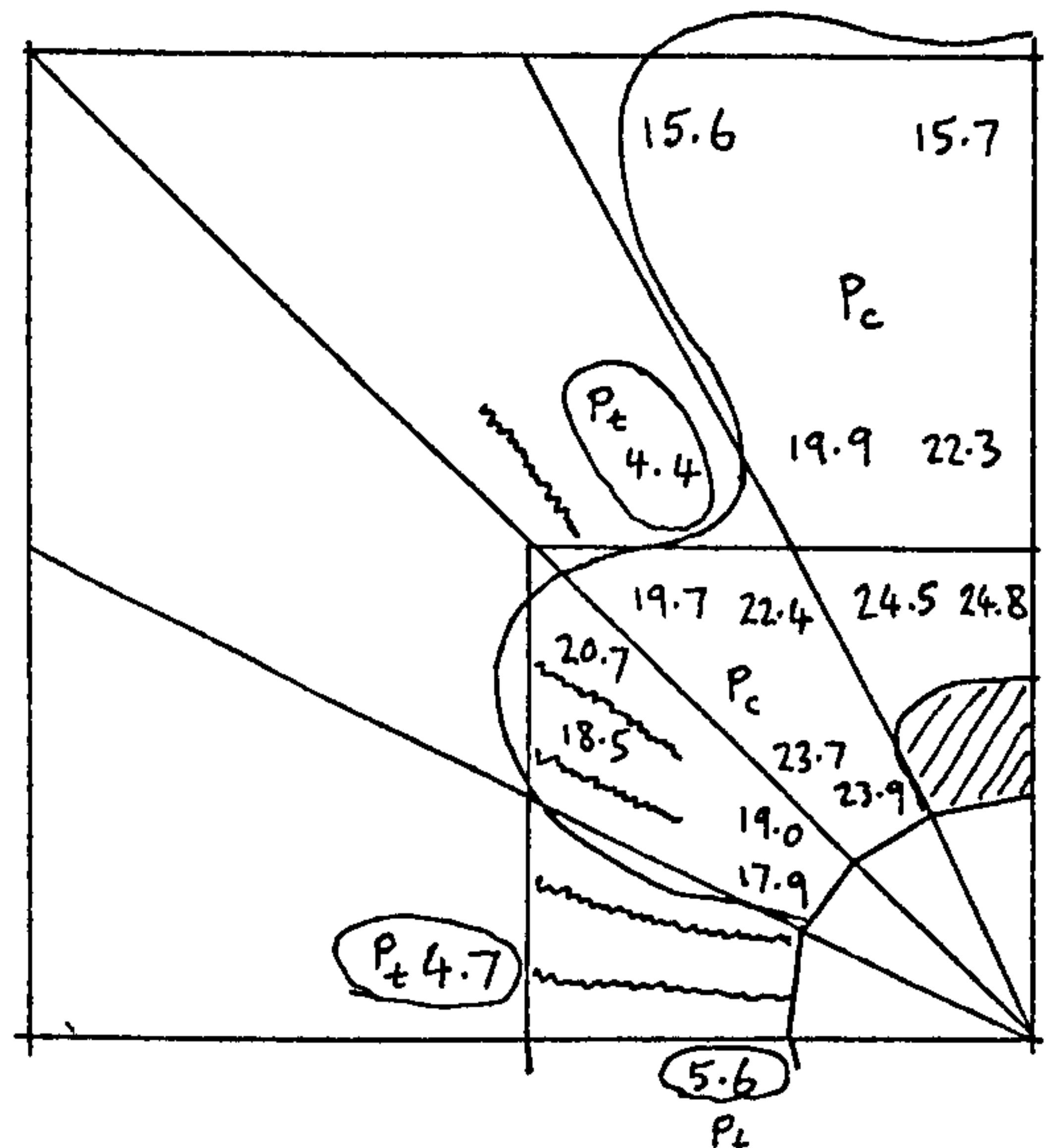
Load step 66
