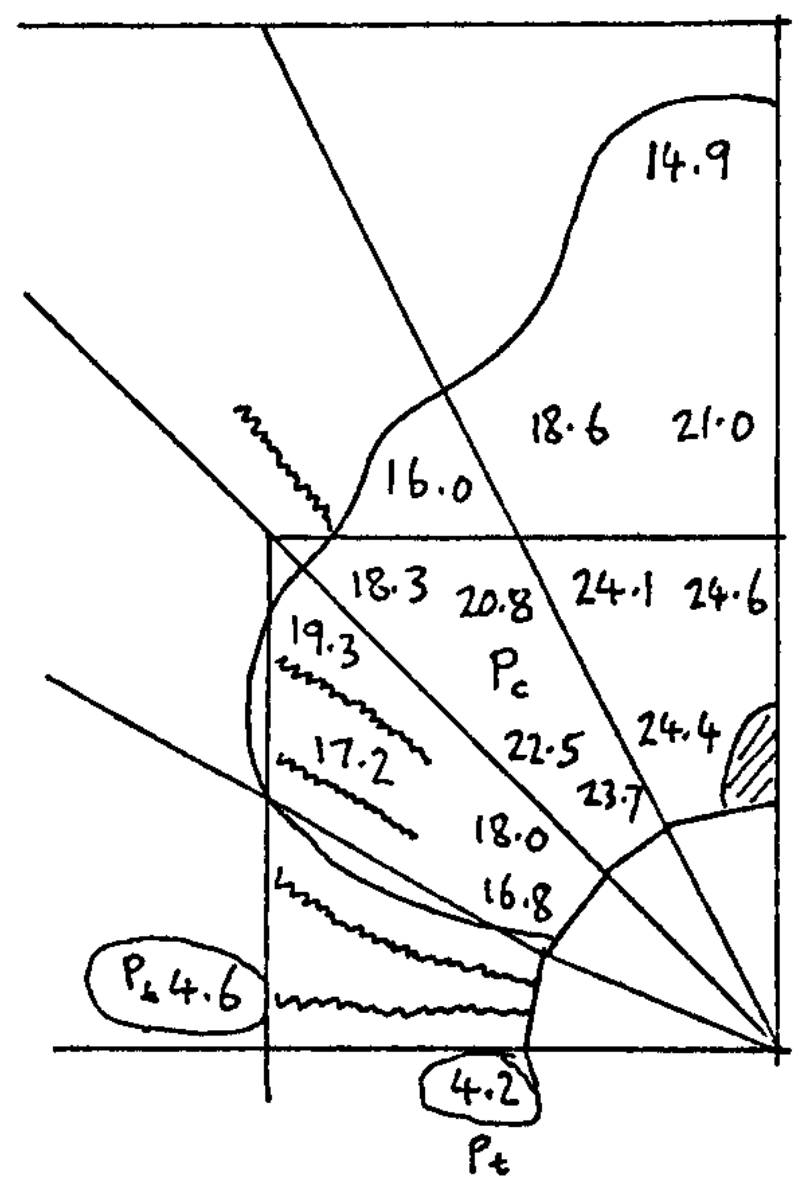
Load step 60
