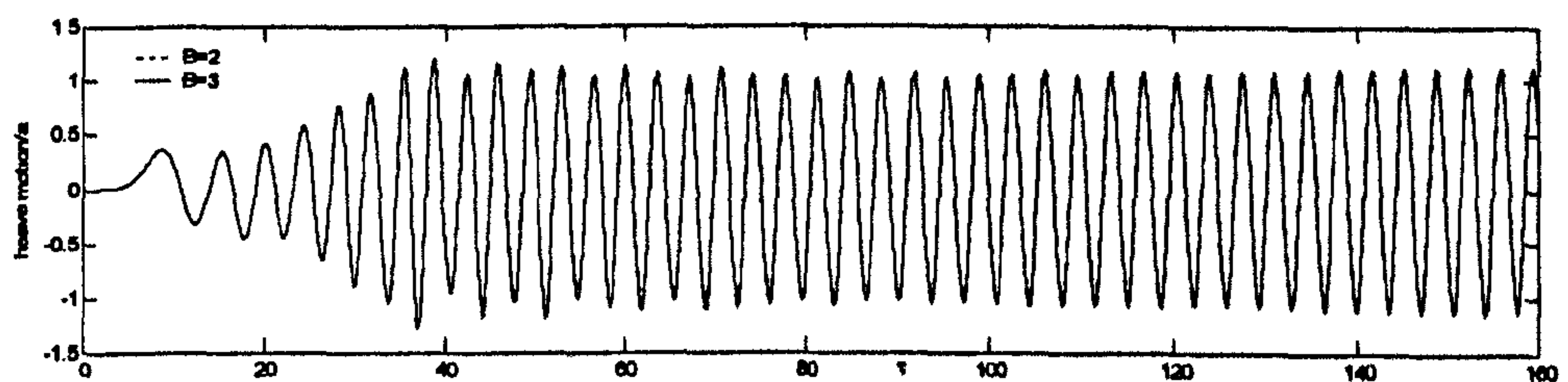
Fig. 9.4.5 (b) heave
