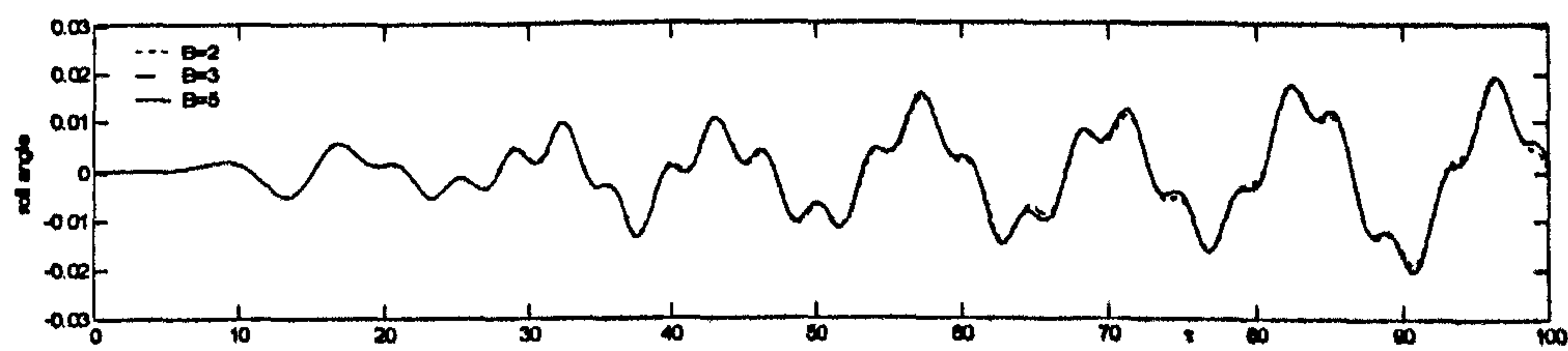
Fig. 9.4.10 (d) roll
