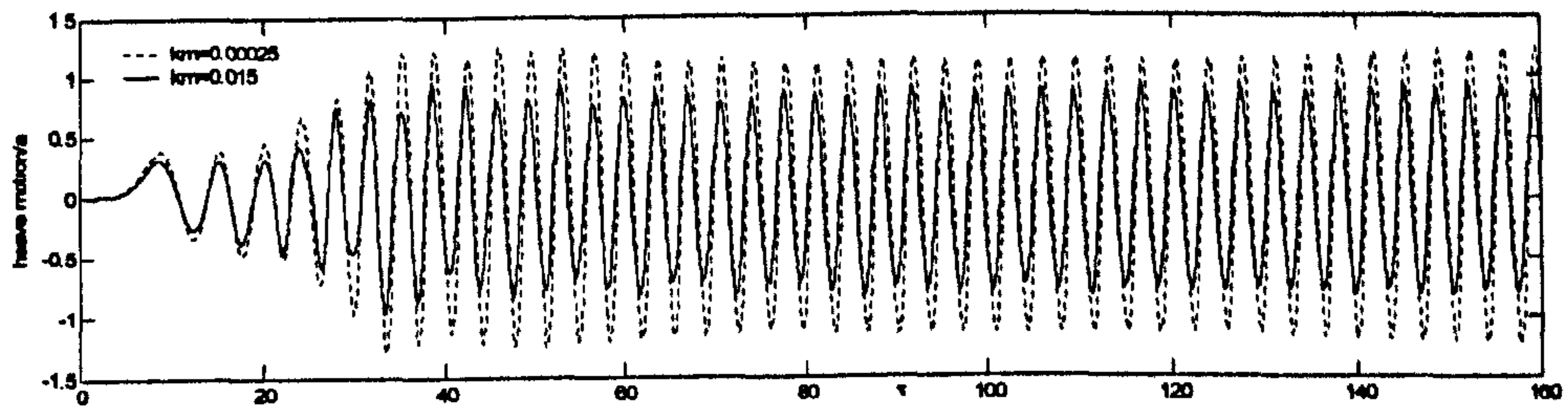
Fig. 9.4.9 (a) heave
